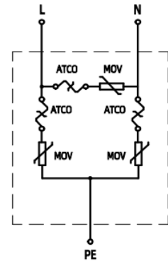
SD05KxxxNM 系列 SD05K-4
