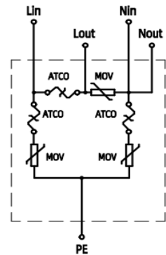
SD05KxxxNMT 系列 SD05K-8
