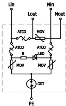
SD05KxxxAMT 系列 SD05K-5
