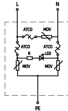
SD05KxxxLM 系列 SD05K-3
